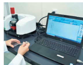
フーリエ変換型赤外分光光度計
